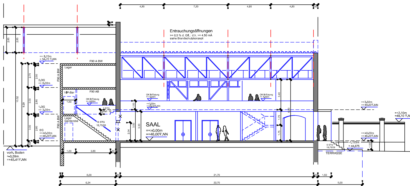
SCHNITT B
